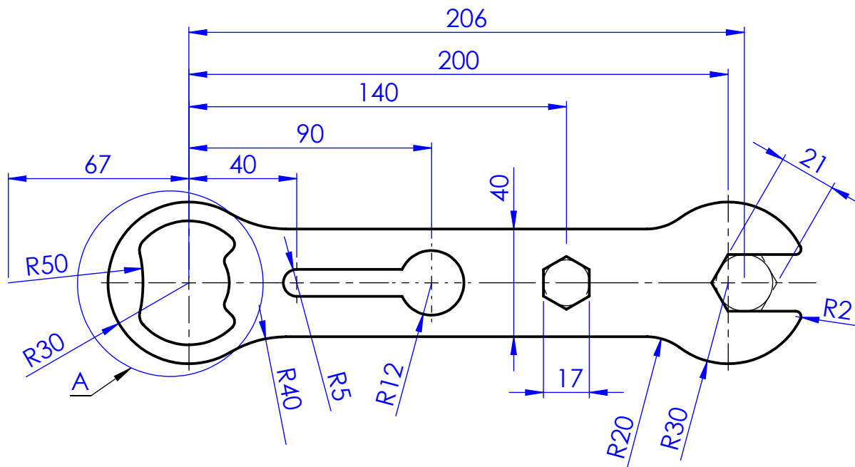
SZCZEGÓŁ A SKALA 1 : 1
